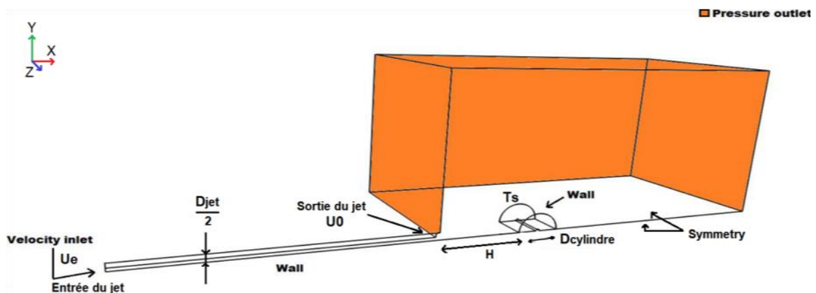
Figure 2: Modèle numérique avec conditions aux limites
